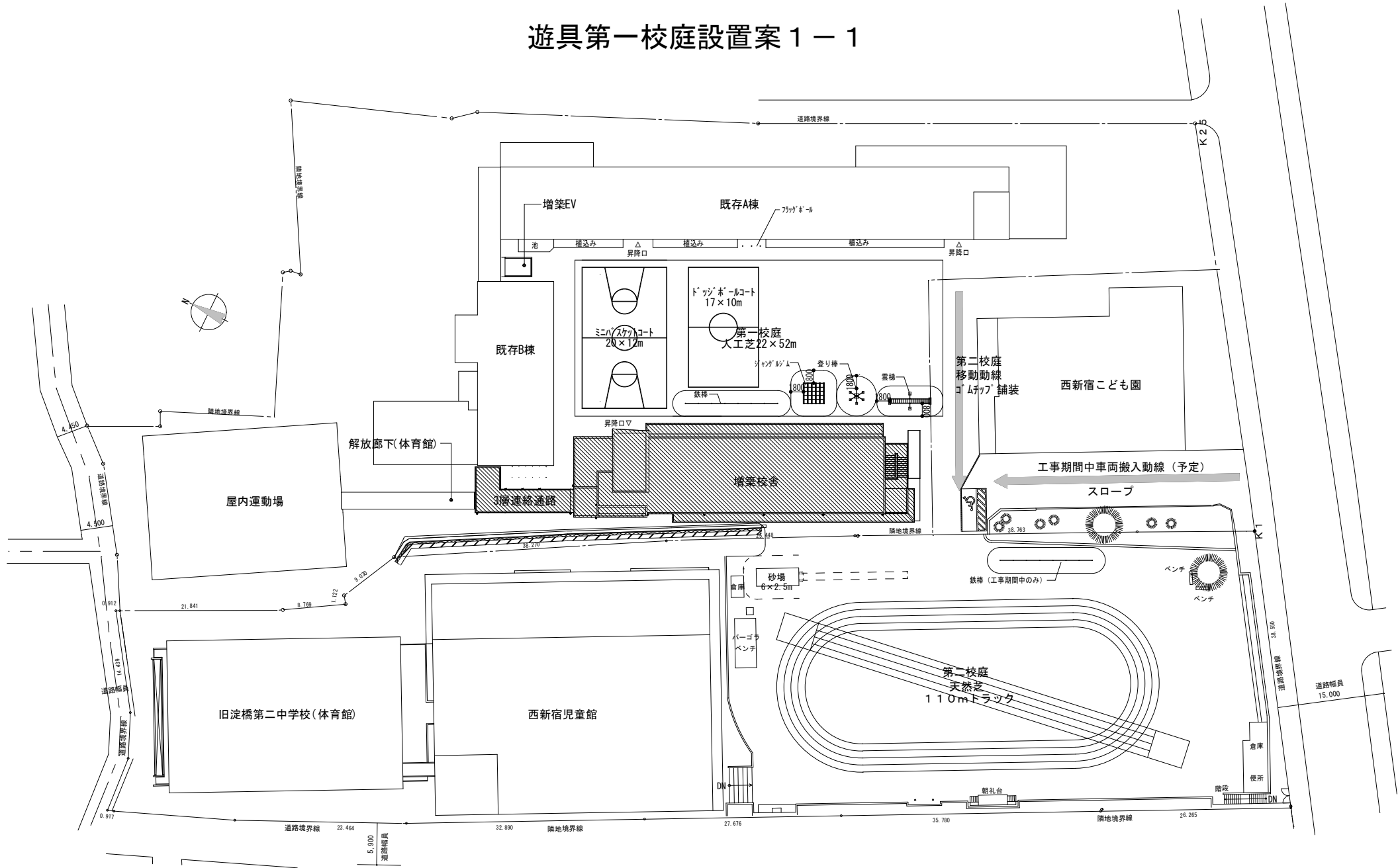
配置図 1 : 500
